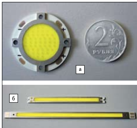
Рис. 3. Светодиодные модули REFOND: а) серия RF-WNCD32DS-5W; б) серии RF-WNL120DS-5W и RF-WNL200DS-10W (1)
