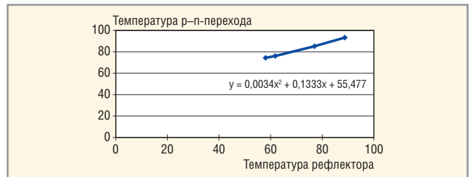
Рис. 4. График зависимости температуры рефлектора от температуры кристалла
